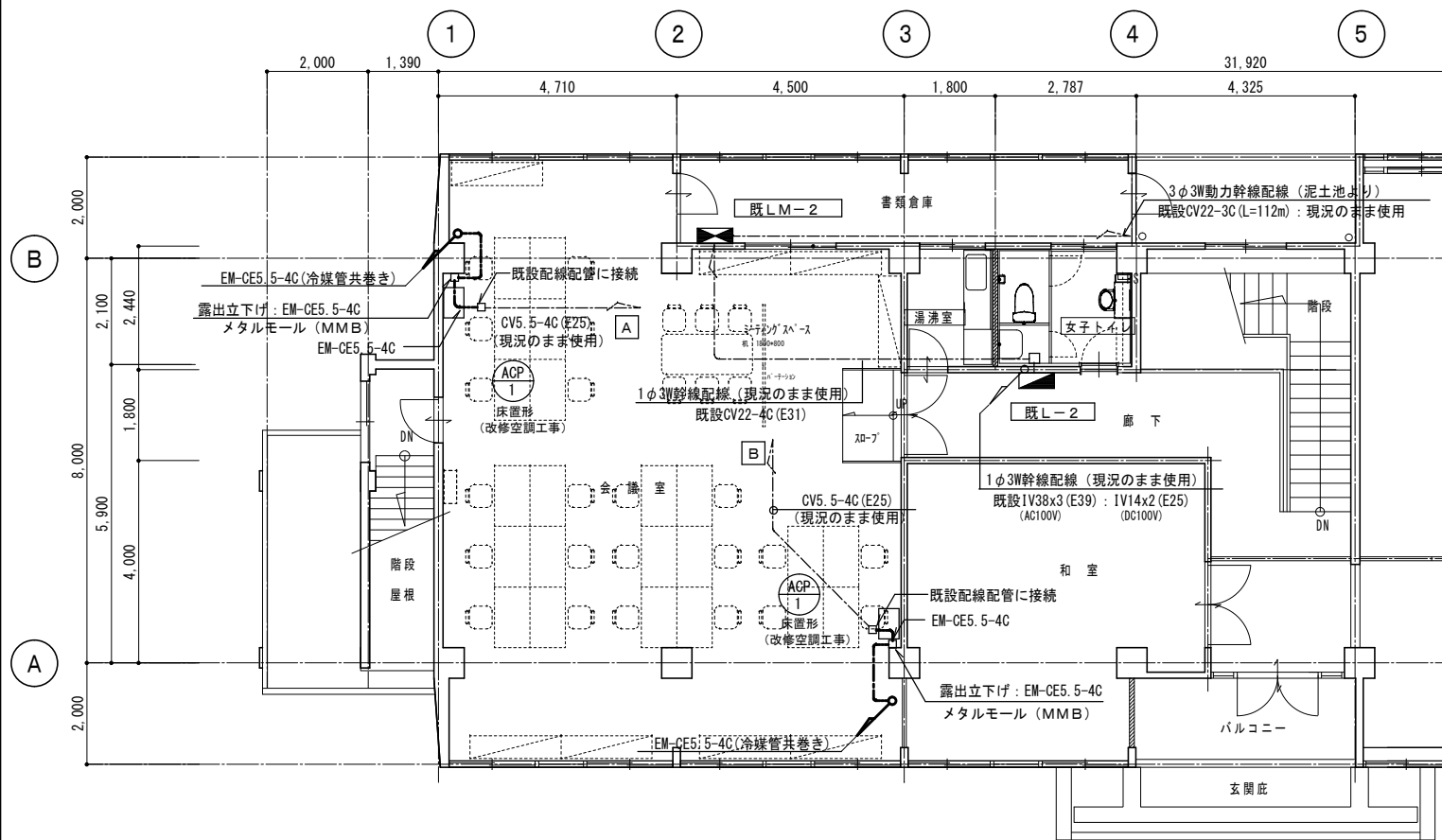
改修 2階平面図 S=1/100 (幹線・動力・盤配線図)
