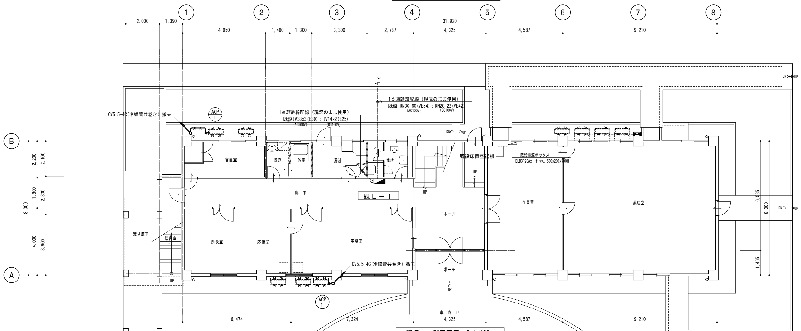
現況 1階平面図 S=1/100
