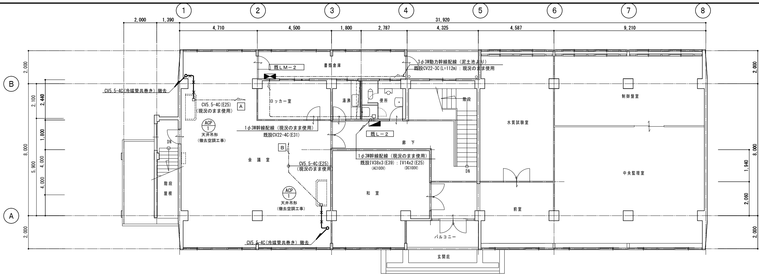
現況 2階平面図 S=1/100
