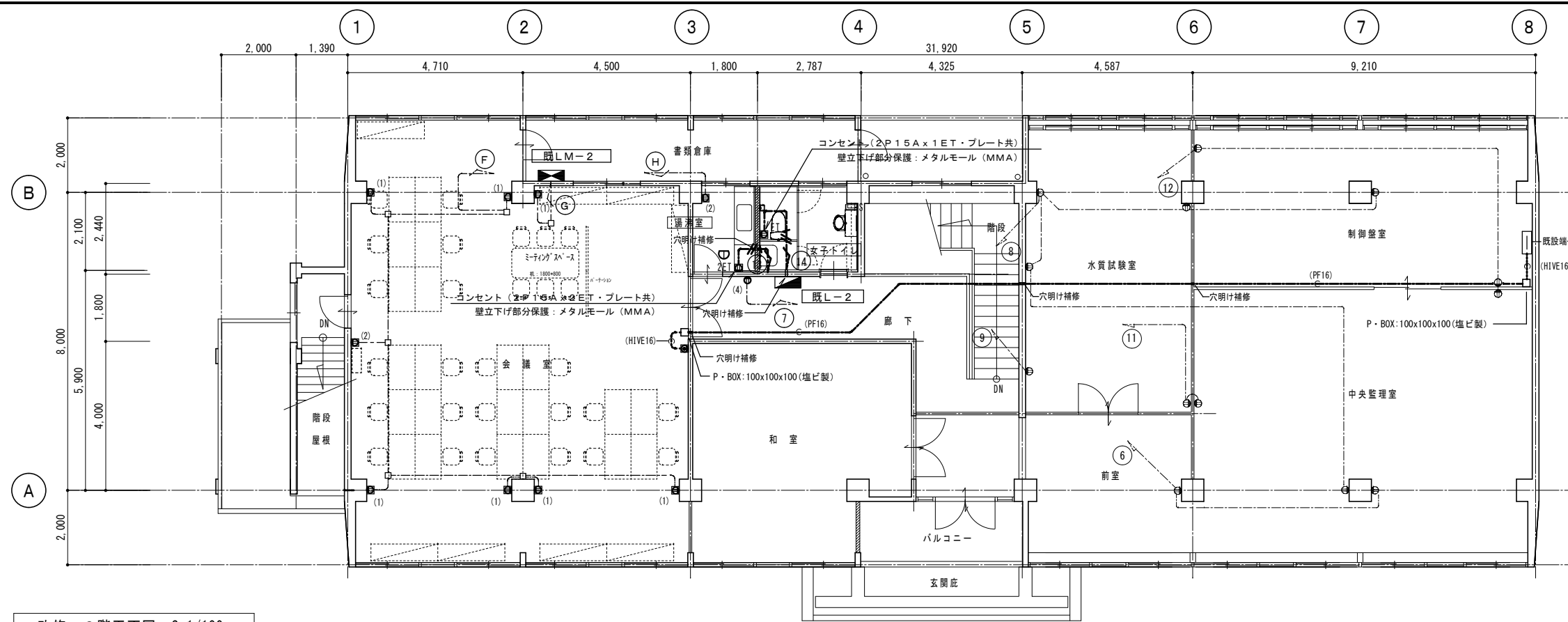
改修 2階平面図 S=1/100
