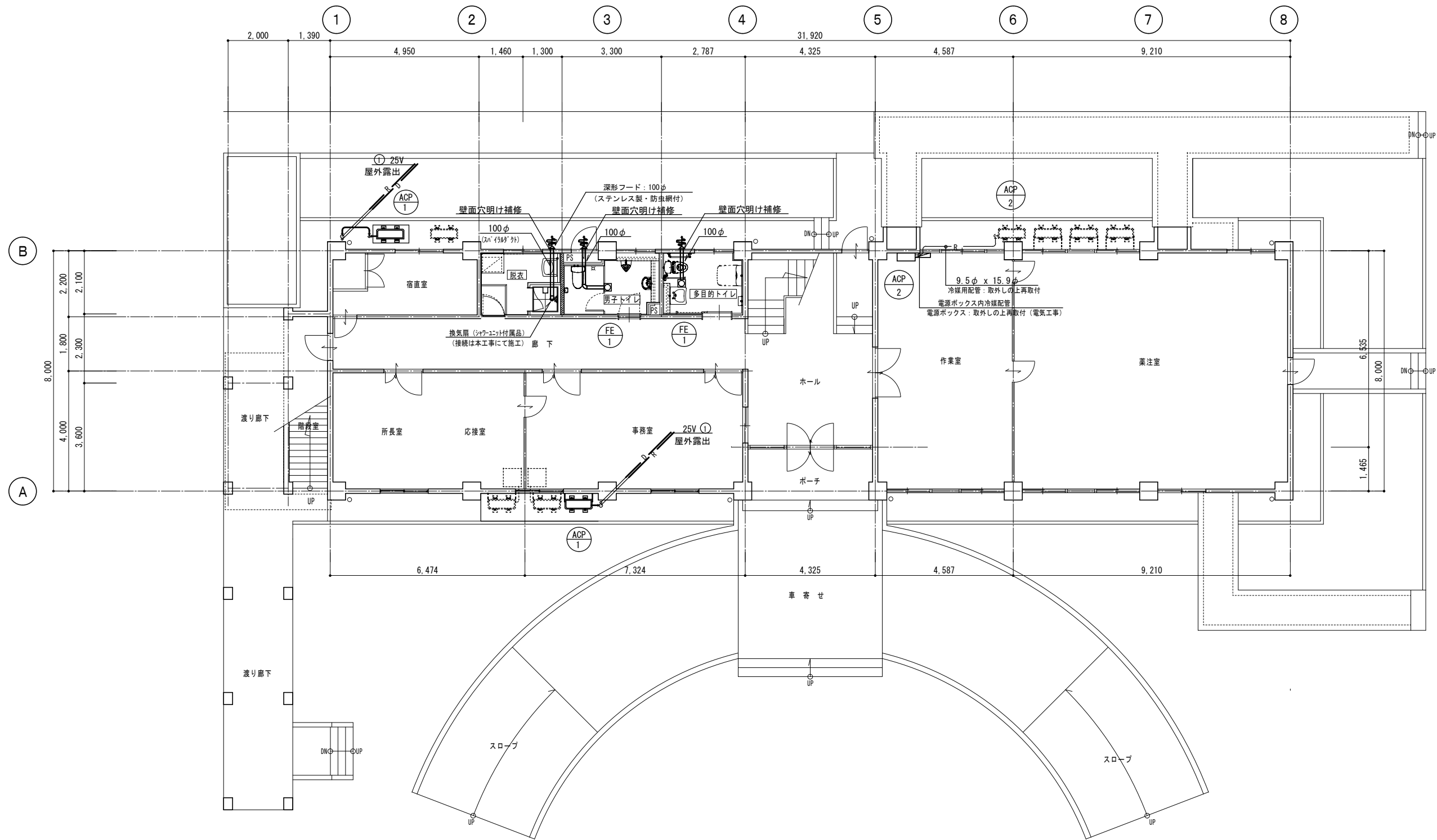
改修 1階平面詳細図 S=1/100
