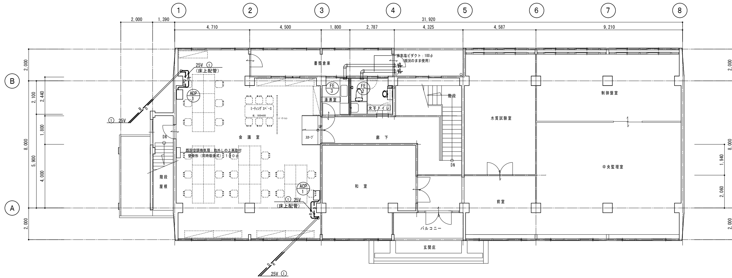
改修 2階平面詳細図 S=1/100
