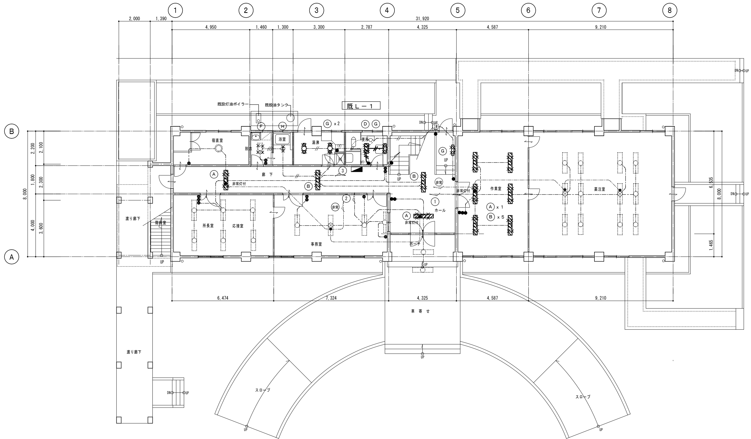
現況 1階平面図 S=1/100
