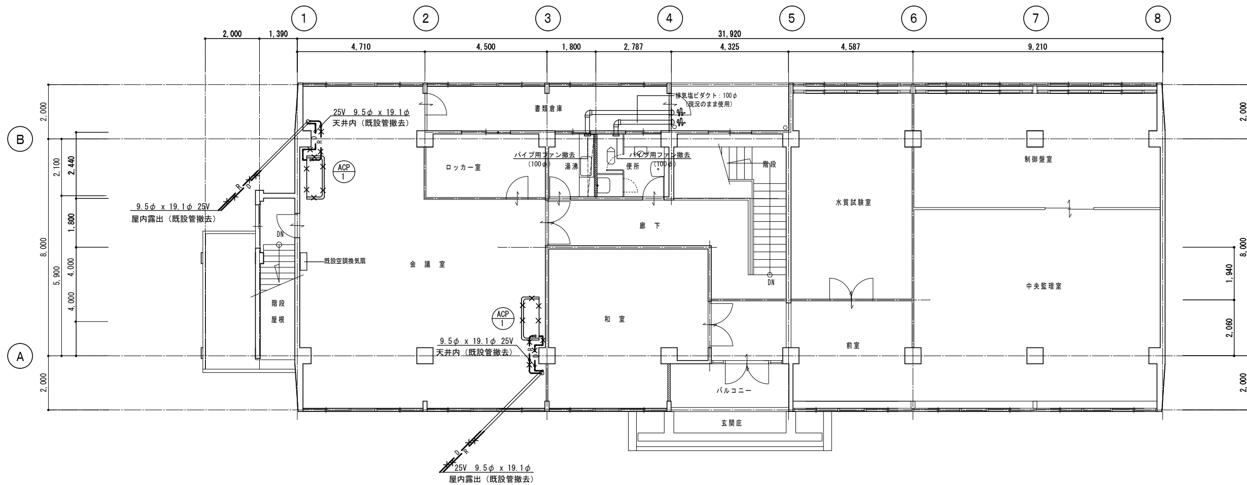
現況・撤去 2階平面詳細図 S=1/100
