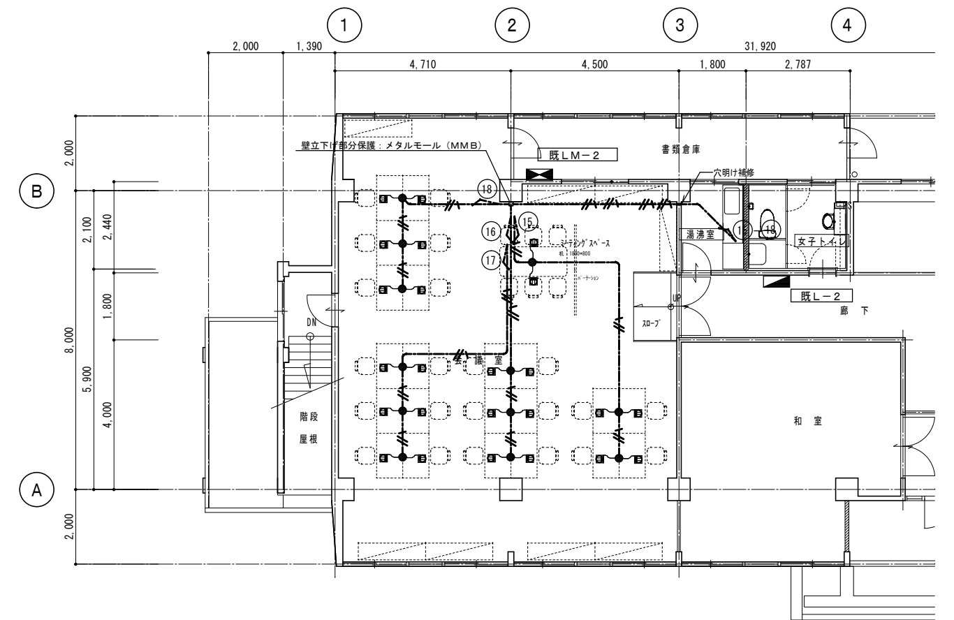
改修 2階平面図 S=1/100 (0Aコンセント配線図)
