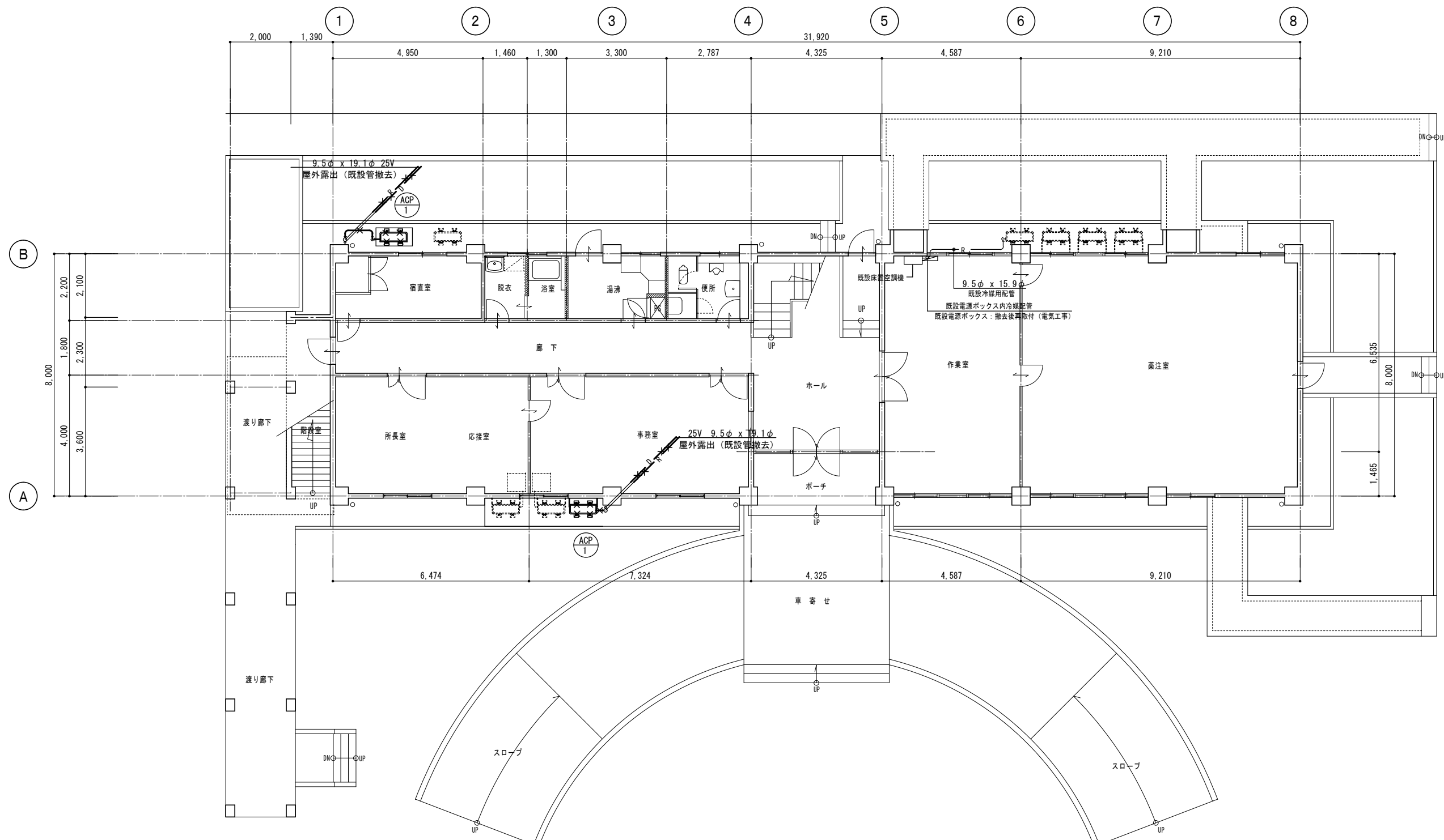
現況・撤去 1階平面詳細図 S=1/100
