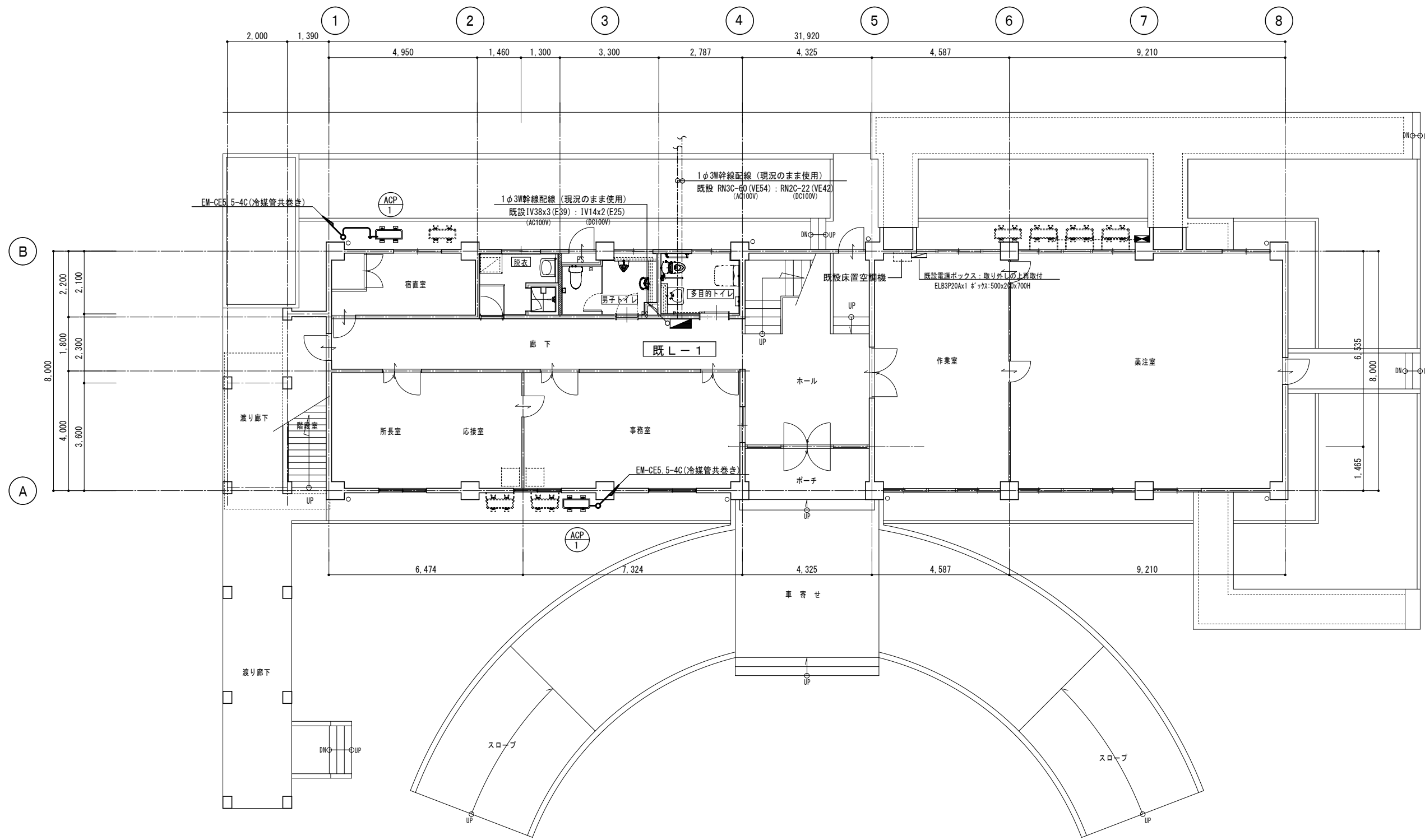
改修 1階平面図 S=1/100
